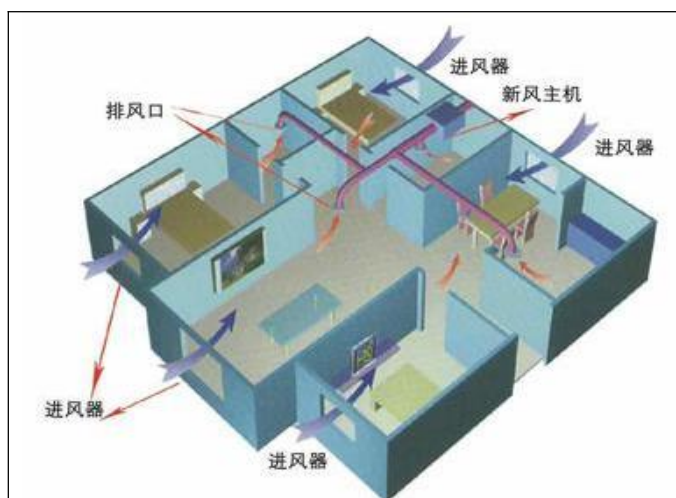
图 4-2 新风系统原理示意图
