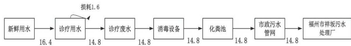
图 2-1 本项目水平衡（t/a）
