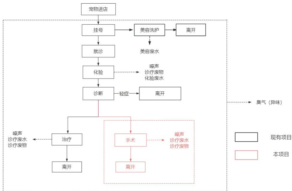
图 2-3 项目诊疗流程及产污环节图
