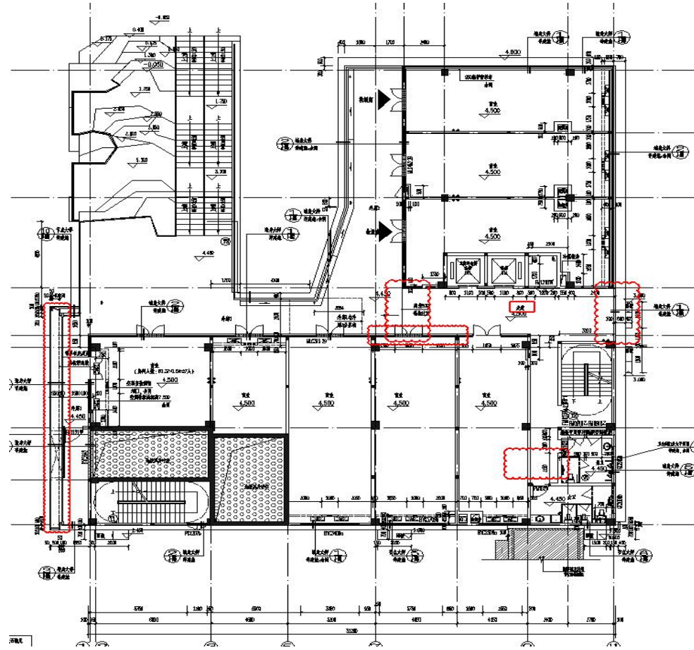
原二层平面图
