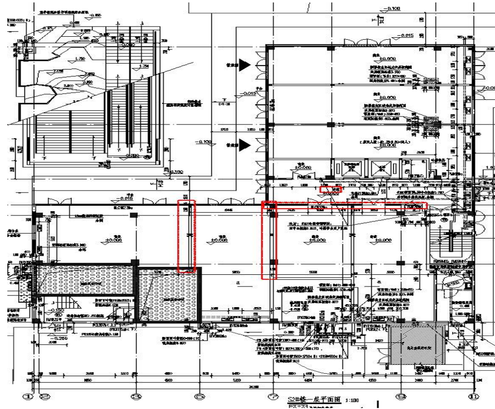
原一层平面图
