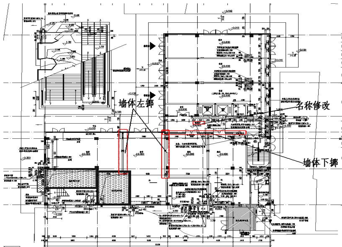
拟调整一层平面图
